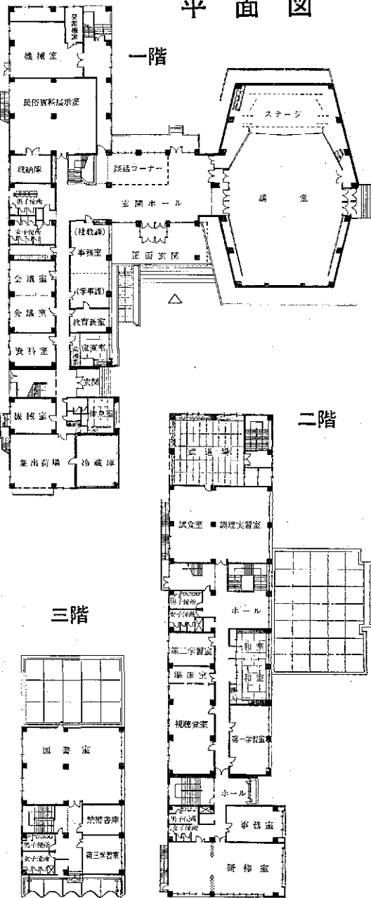
平面図
